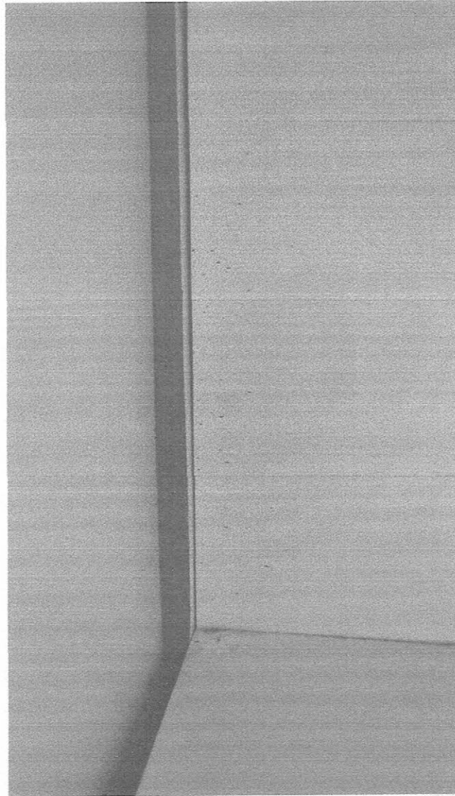
Figura 10 - Estufamento, descolamento, empenamento e presença de mofo na estrutura do móvel.
