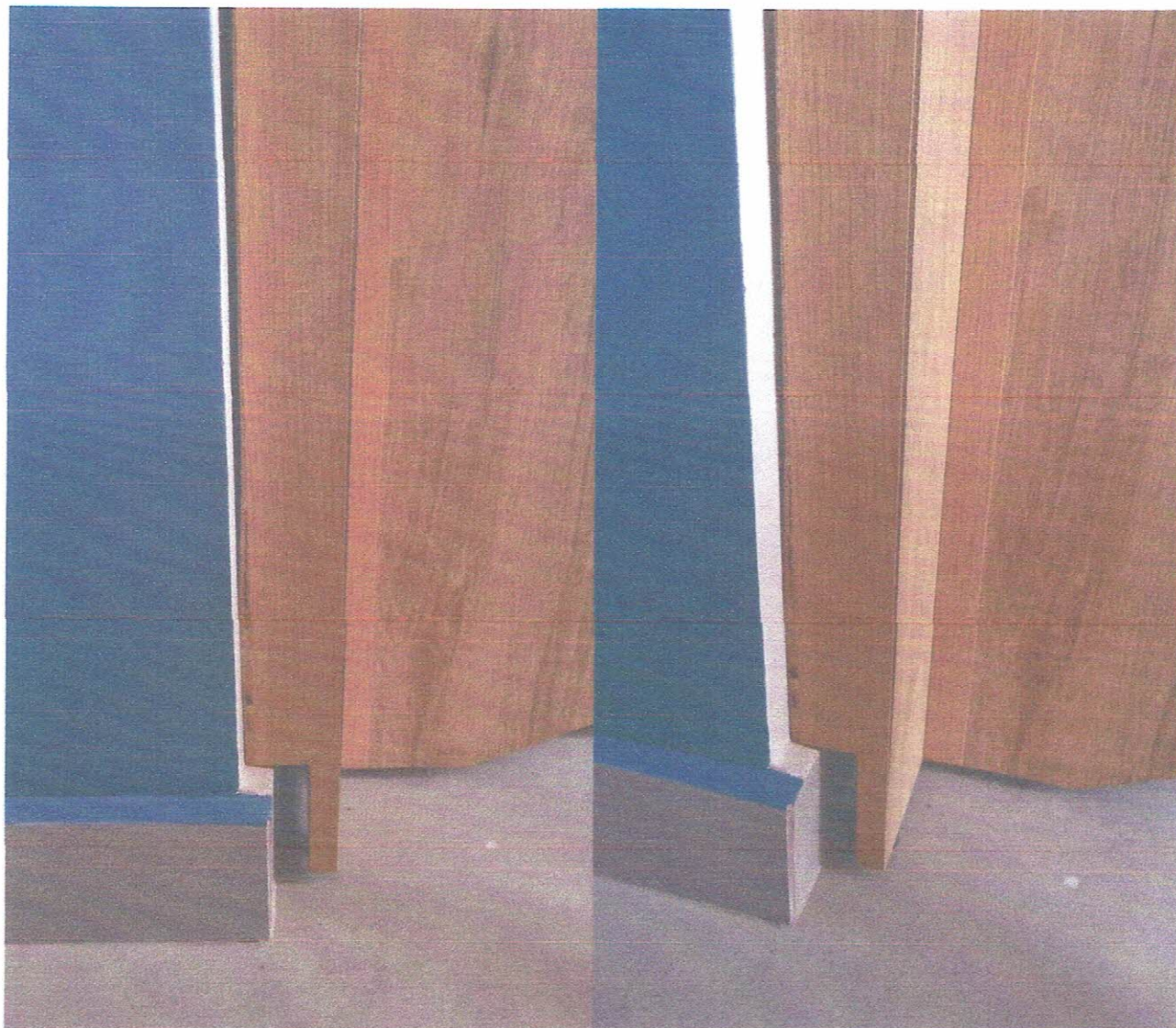
Figura 4 - Estufamento, descolamento, empenamento e presença de mofo na estrutura do móvel.
